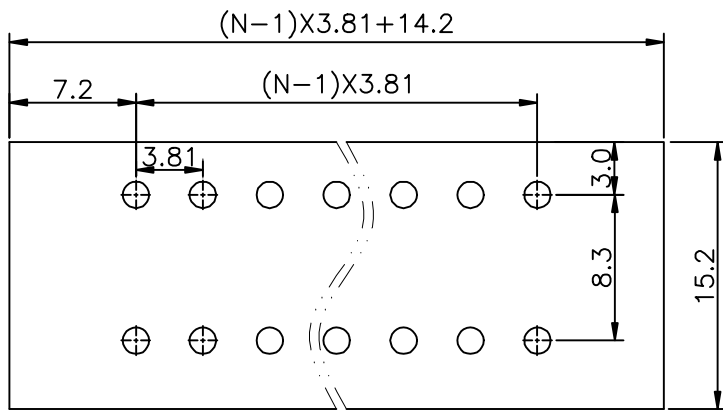
P.C.B. LAYOUT
