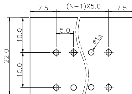
PCB LAYOUT( \pm 0.05 )
