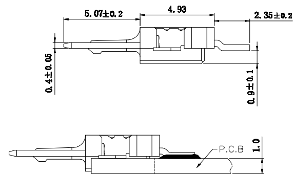
PCB寸法 (T=1.0mm) PCB Layout (T=1.0mm)
