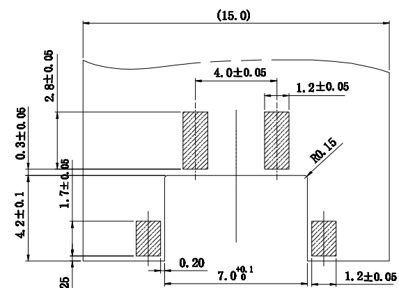
PCB寸法 (T=1.0mm) PCB Layout (T=1.0mm)
