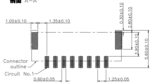
PCB寸法 PCB Layout
