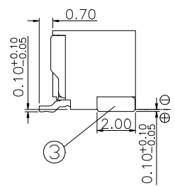
剖面 A-A
