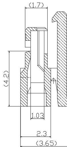
SECTION A-A
