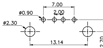
PCB LAYOUT(±0.05)
