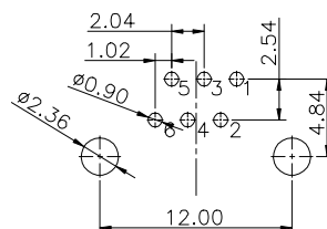
PCB LAYOUT(±0.05)
