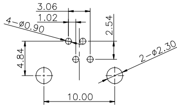
PCB LAYOUT(±0.05)
