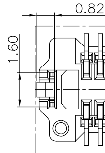
DETAIL B 2:1
