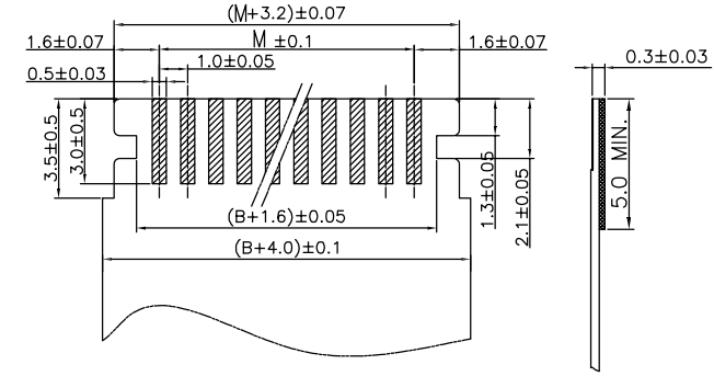
适用FPC寸法 APPLICABLE FPC
