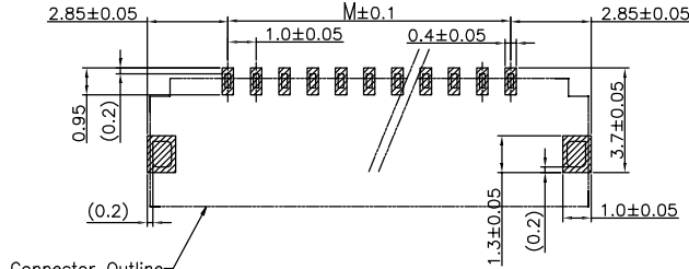
适用PCB布局 RECOMMENDED PCB LAYOUT
