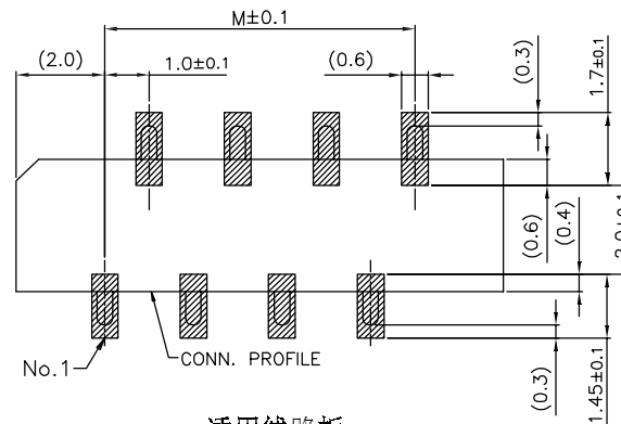
适用线路板 RECOMMENDED PCB LAYOUT
