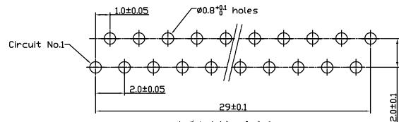
适用线路板 RECOMMENDED PCB LAYOUT
