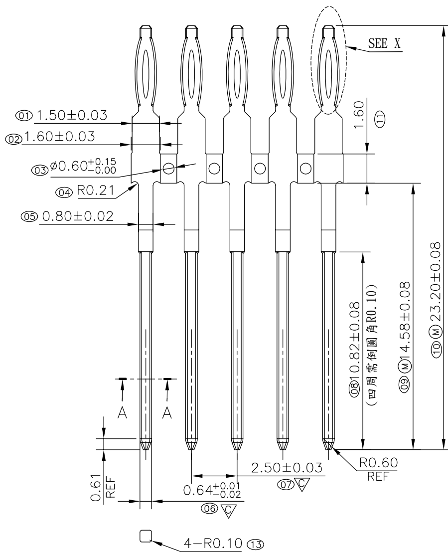
SECTION A-A
